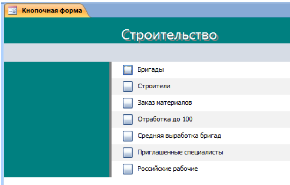
Рис 4.3 Кнопочная форма
